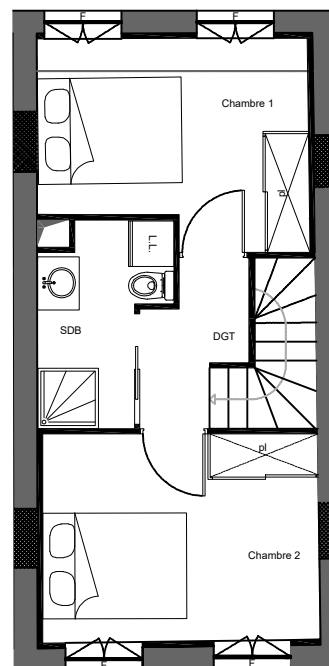
Niveau R+1
